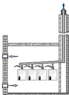
Система каскадного дымоотведения забор воздуха из помещения
