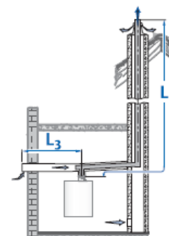
GAL-K в канале, забор воздуха снаружи
