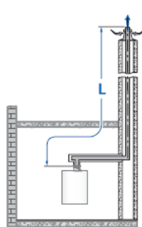
GA-K забор воздуха из канала
