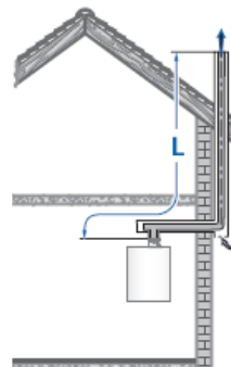
GAF-K по фасаду, забор воздуха снаружи
