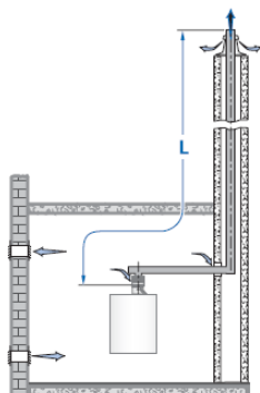
GA забор воздуха из помещения
